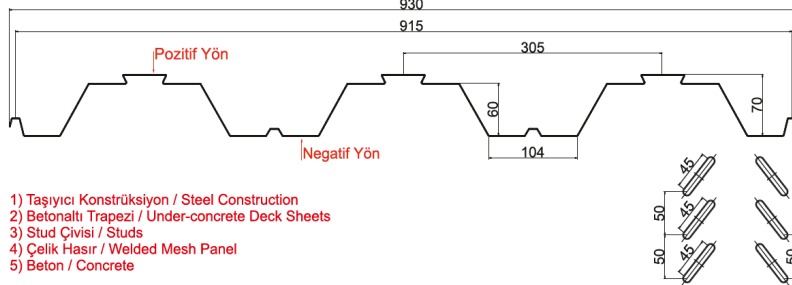
Ölçü çizimi — tüm ölçüler mm
